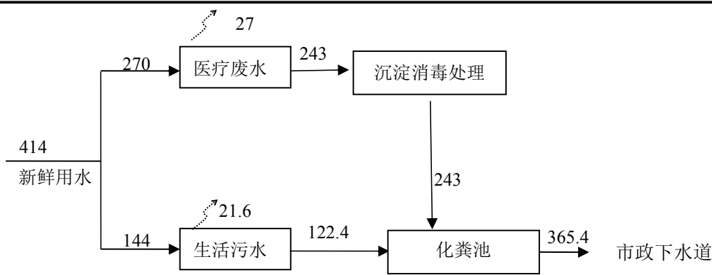
项目水平衡图 (单位: t/a)
